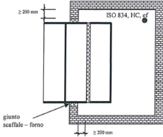
Fig. 1: PIANTA
