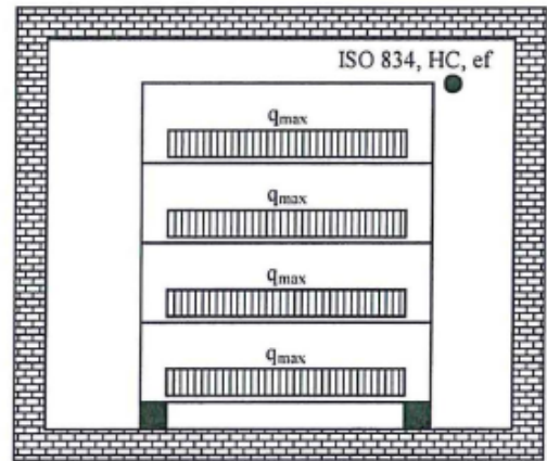
Fig. 5: SEZIONE VERTICALE
