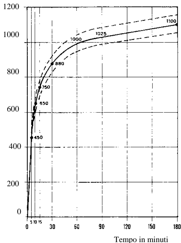
Fig. 2 – Curva temperatura - tempo.
